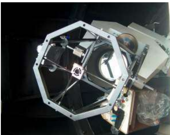
Das neue Newton-Teleskop. Links: Blick von vorne auf den Hauptspiegel. Rechts: Blick zum Fangspiegel und auf die beiden Ausgänge.
